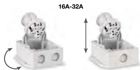
Tipo TOP: base reversible y toma extraíble para un cableado fácil y flexibilidad para la entrada de cable.
